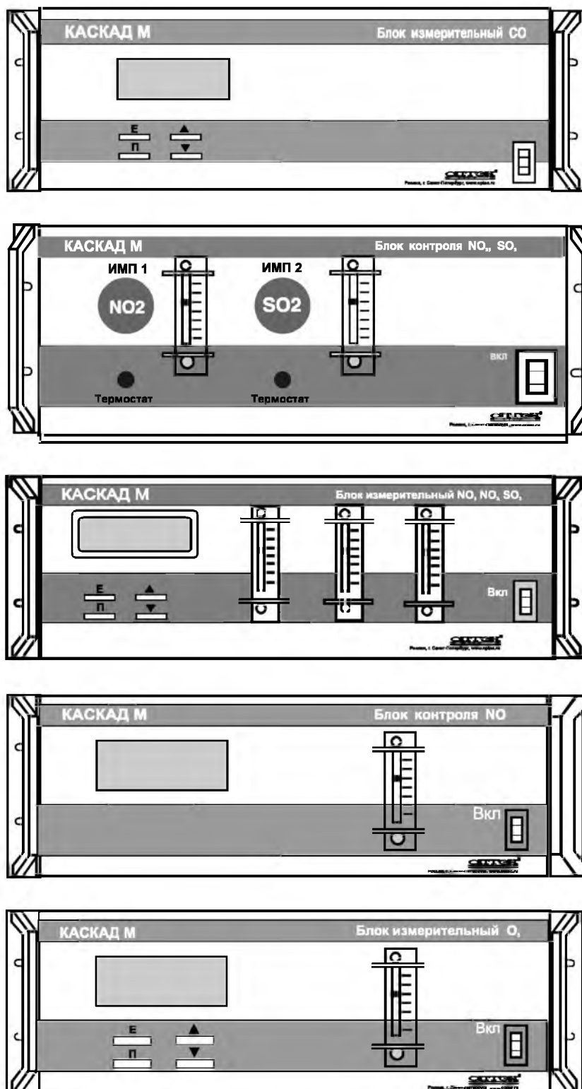
Рисунок 1 – Внешний вид газоанализатора КАСКАД-М.
